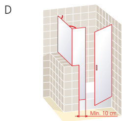
Frontal 1 puerta con 1 fijo a continuación con forma adaptada y 1 fijo en ángulo sobre tabique
