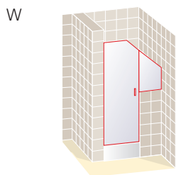
Frontal 1 puerta con 1 fijo a continuación sobre tabique, ambos con forma adaptada
