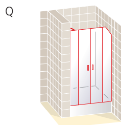
Frontal 2 puertas con 2 fijos a continuación, uno de ellos con forma adaptada
